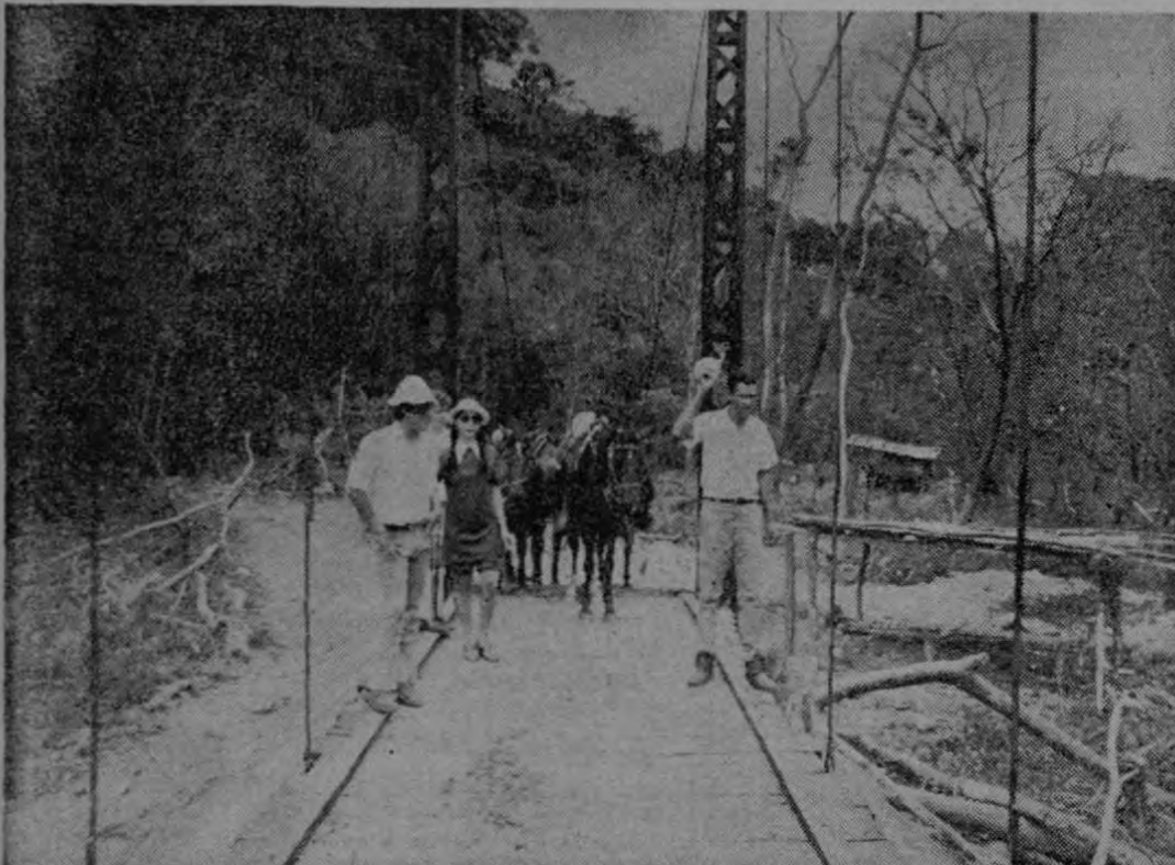
Este es el puente sobre la Quebrada Cedros, Buenos Aires y Salitre. Con este puente se habilita una vasta y rica zona agrícola.
